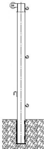
Fig 3. Stalpul de tenis in pozitia montat.
