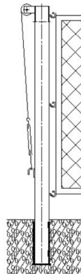
Fig 4. Stalpul de tenis in pozitia montat, inclusiv fileul.
